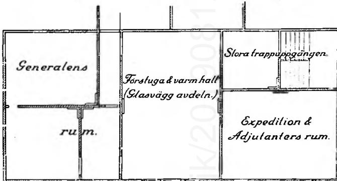
Nedre våningen.
