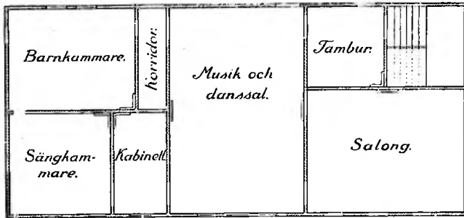
Öfre våningen.
